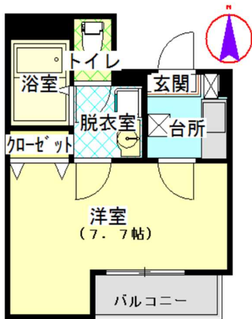
101号室間取り
